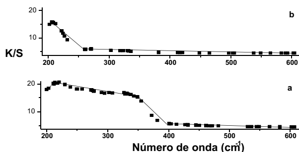
Fig. 4. Espectro de reflectância difusa no UV-Vis da (a) fibra de PVA/TiO 2 (5% m/m) e da (b) fibra de PVA.
