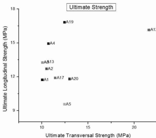
Fig. 3. Resistência à tração das palhas de milho estudadas nos sentidos longitudinal e transversal.
