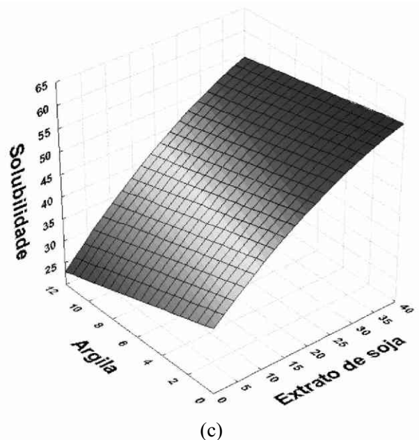
Fig. 1. Efeito da argila e do extrato de soja sobre a espessura (a), permeabilidade ao vapor de água (b) e solubilidade em água dos filmes(c).
